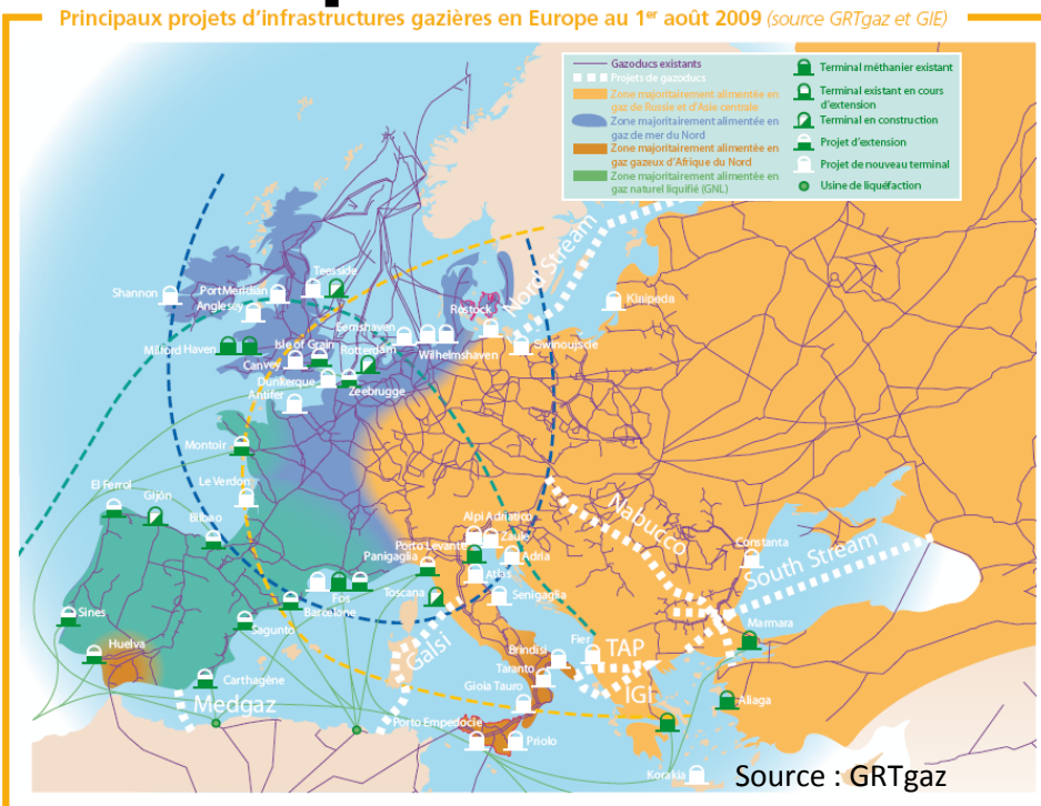
Principaux projets d'infrastructures gazières en Europe au 1 er août 2009 (source GRTgaz et GIE)
